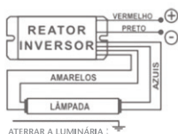
Esquema de ligação
